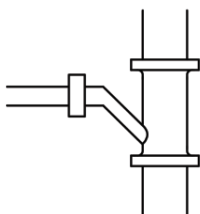
Соединение дренажных труб с помощью тройника
