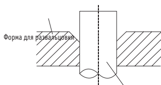
Рис. 7.7 Труба
