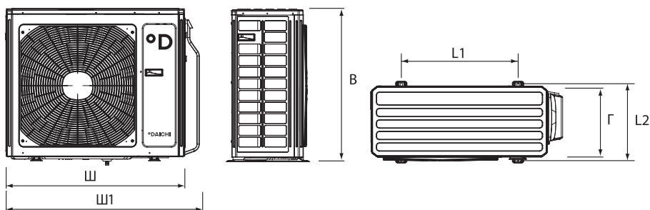
ГАБАРИТЫ, ММ
