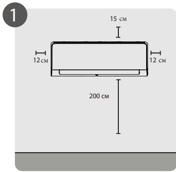
1 Выбрать место для установки
