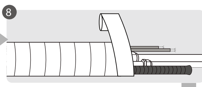
8 Обвяжите трубопроводы и кабели
